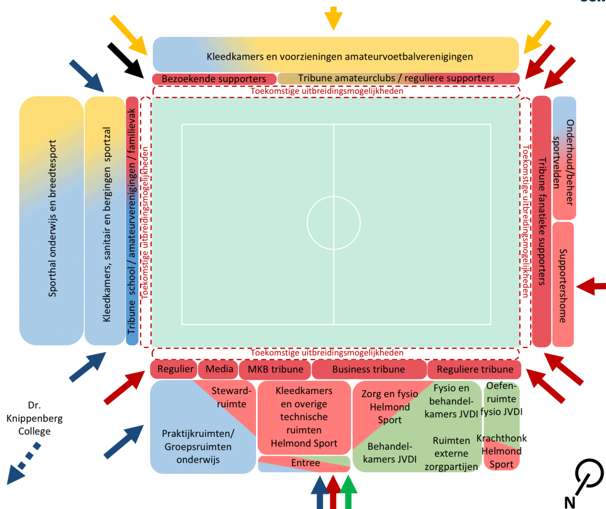
Figuur 3.3 Laag 1 (begane grond) – Vleckenplan/concept indeling van de MFSA
